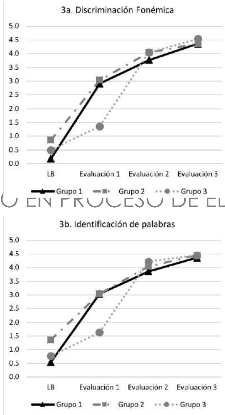
Gráfica 3. Promedio de puntuaciones de sensibilidad a la segmentación a lo largo del tiempo
