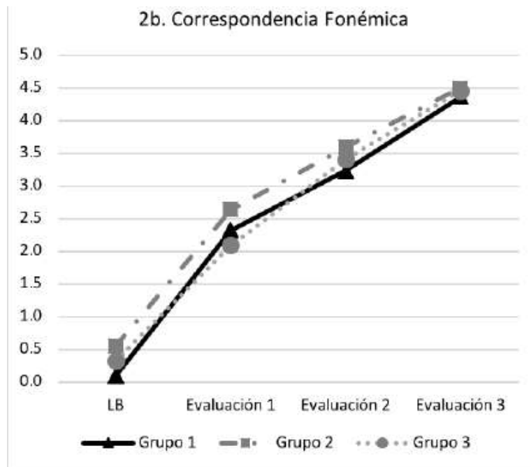
Gráfica 2. Promedio de puntuaciones de sensibilidad a la rima a lo largo del tiempo.
