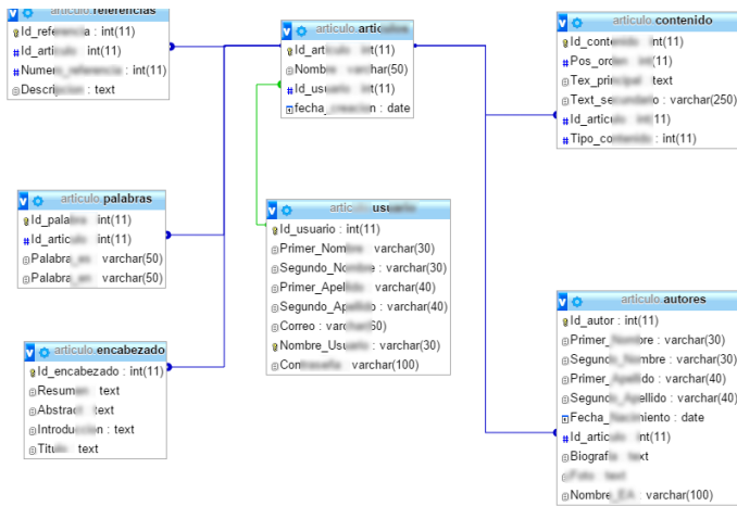
Figura 4. Diseño MER de la base de datos de la aplicación web
