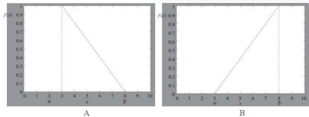
Figura 2. Función tipo saturación A. Derecha B. Izquierda
