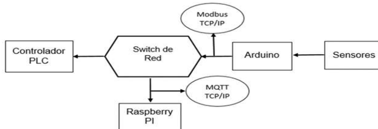
Figura 1. Estructura de la comunicación entre el PLC y Arduino
