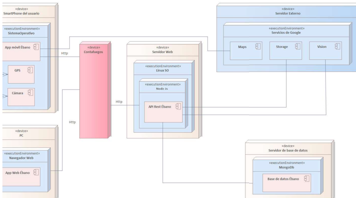
Figura 7. Vista Física
